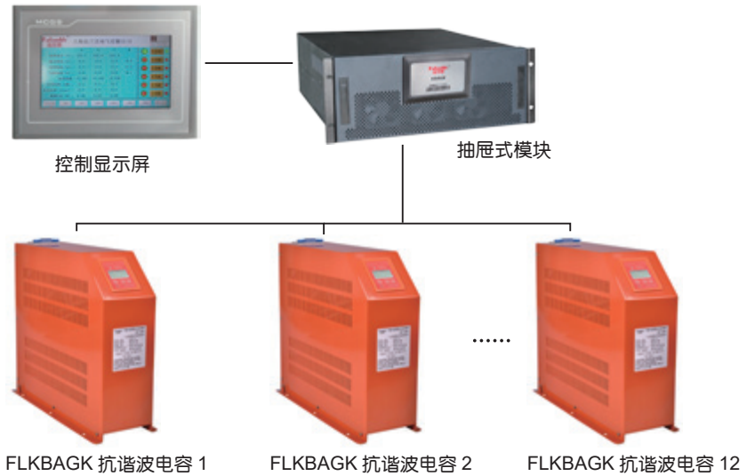
FLKAPFC 或 FLKSVG C 结构示意图
